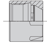
ER 11, 16, 20, 25 Mini
